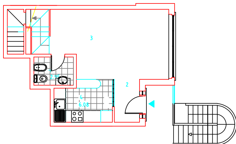
1º ANDAR
