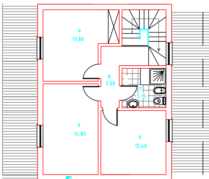
2º ANDAR
